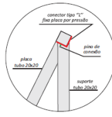
VISÃO LATERAL DO CAVALETE - 50 x 110 cm
